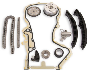
凸轮轴链套件
